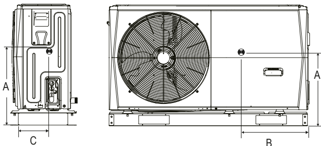
4/6 kW (dimenzije v mm)
