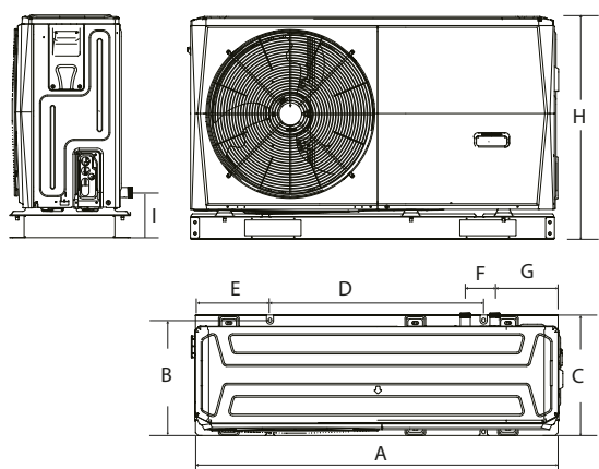
4/6 kW (dimenzije v mm)
